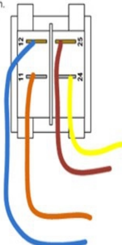
SW-491 Switch
